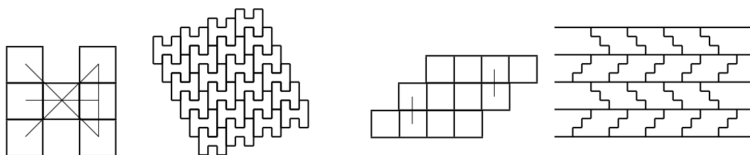
A Shannon-Pollak parkettázás.
