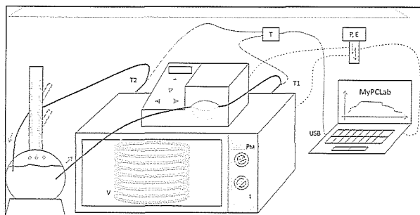
1. ábra: Kísérleti berendezés
