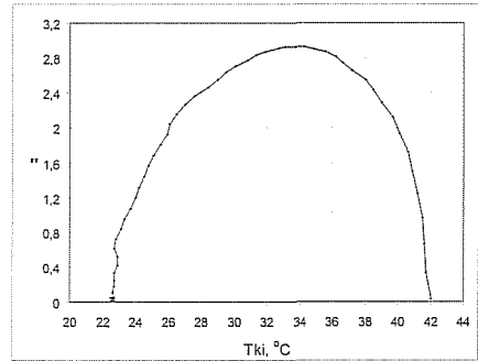
2. ábra: \varepsilon'' a kimeneti hőmérséklet függvényében napraforgó olaj mikrohullámú átészterezése során
