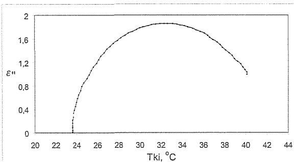
3. ábra \varepsilon'' a kimeneti hőmérséklet függvényében repceolaj mikrohullámú átészterezése során
