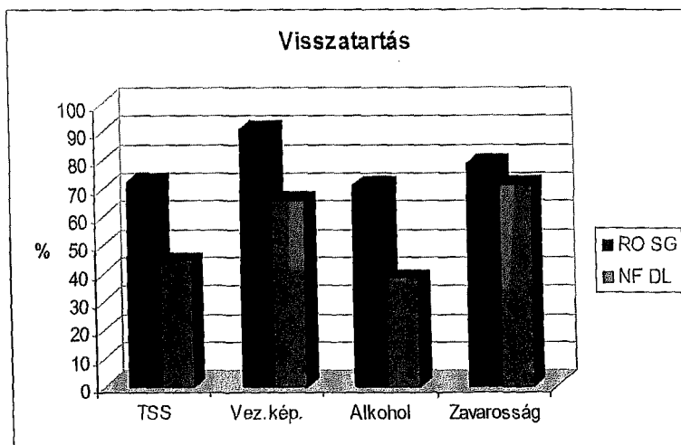
5. ábra: Jellemző komponensek visszatartási értékei a bor reverz ozmózis (RO) és nanoszűrése (NF) esetén.
