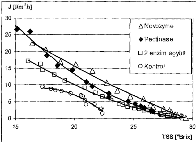
6. ábra: A különböző enzimes előkezelés hatása a fluxus értékére gyümölcslevek sűrítésénél
