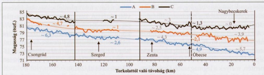
4. ábra – Az ártéri szintek magasságának és esésének változása Csongrád és a torkolat között
