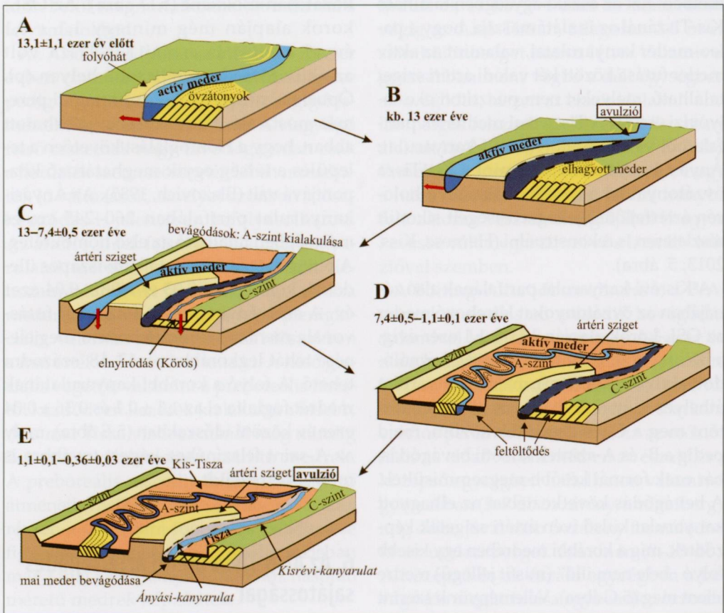
5. ábra – Az északi egység Mindszent–Ópusztaszer közötti szakaszának fejlődéstörténeti vázlata a késő glaciálstól napjainkig
