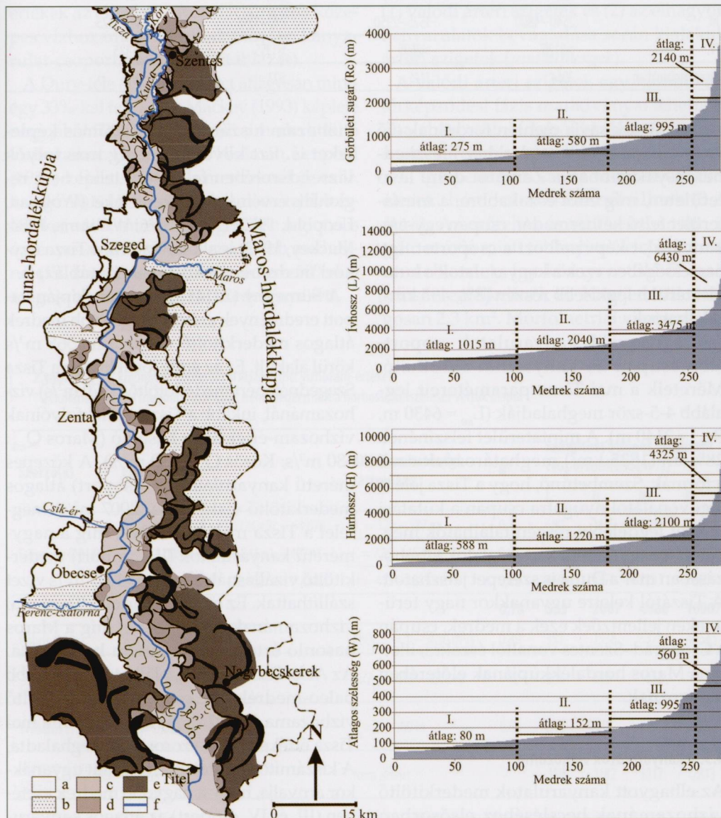
2. ábra – A különböző morfológiai csoportokba tartozó kanyarulatok előfordulása és az egyes csoportokhoz tartozó átlagos morfológiai paraméterek
