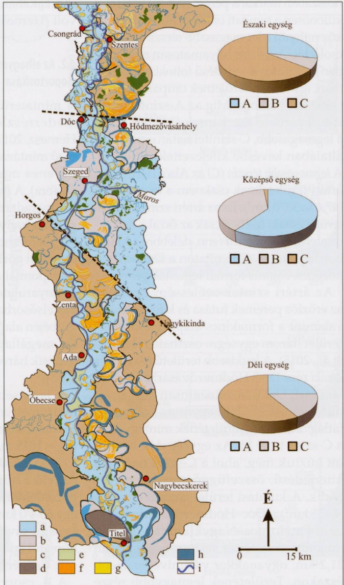
1. ábra – A kutatási terület geomorfológiai térképe az elkülönített morfológiai egységek határaival, valamint az ártéri szintek egységenkénti területarányával a. A-szint; b. B-szint; c. C-szint; d. Titeli-lőszfennsík; e. hullámtér; f. övzátont; g. sarló-lapos; h. elhagyott kanyarulat; i. aktív folyó
