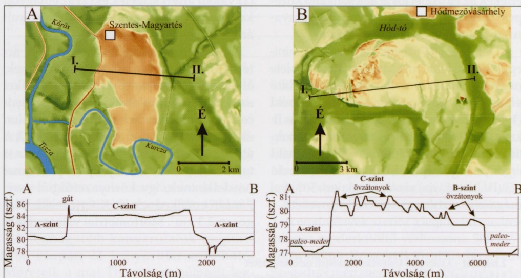
3. ábra – A Szentés–Magyartés mellett található valódi ártéri sziget (A), valamint a Hód-tó kanyarlata által formált umlaufberg domborzata és keresztmetszéne (alaptérkép: 1: 10000)
