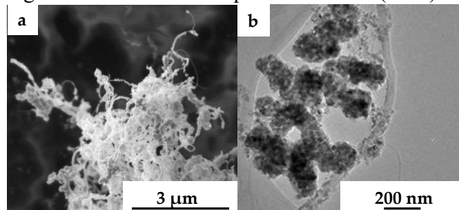
2. ábra Az PE-TiO 2 -WO 3 -700 1:18:1 arányú kompozit SEM (a) és TEM (b) felvétele
