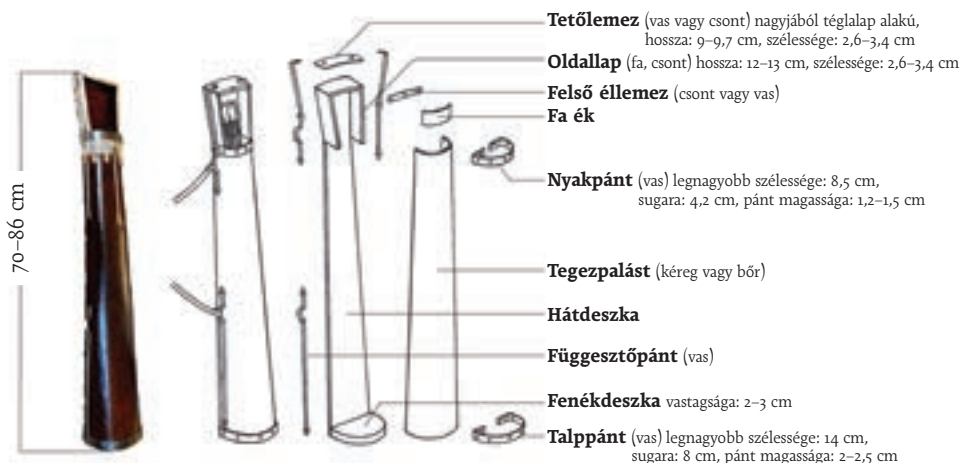
REKONSTRUÁLT HONFOGLALÁS KORI TEGEZ ALKATRÉSZEI ÉS JELLEMZŐ MÉRETEI.
