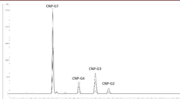
3. ábra A különböző időpontokban injektált minták kromatogramja
