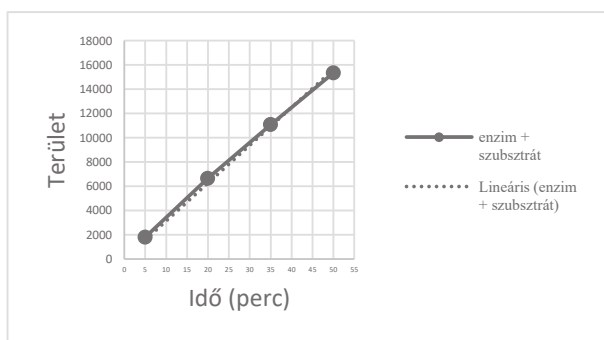
4. ábra A CNP-G3 képződés reakciósebességének meghatározása a CNP-G7-HSA katalizálta hidrolízis reakcióban
