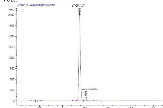
1. ábra Tisztított CNP-G7 szubsztrát HPLC kromatogramja
