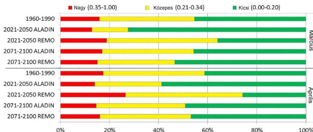
4. ábra. A szélerózió érzékenységi kategóriák kiterjedése (% a mezőgazdasági területek kiterjedéséhez viszonyítva) 1961-1990, 2021-2050 és 2071-2100 közötti időszakban, az ALADIN és a REMO regionális klíma modell szimulációk adatai alapján
