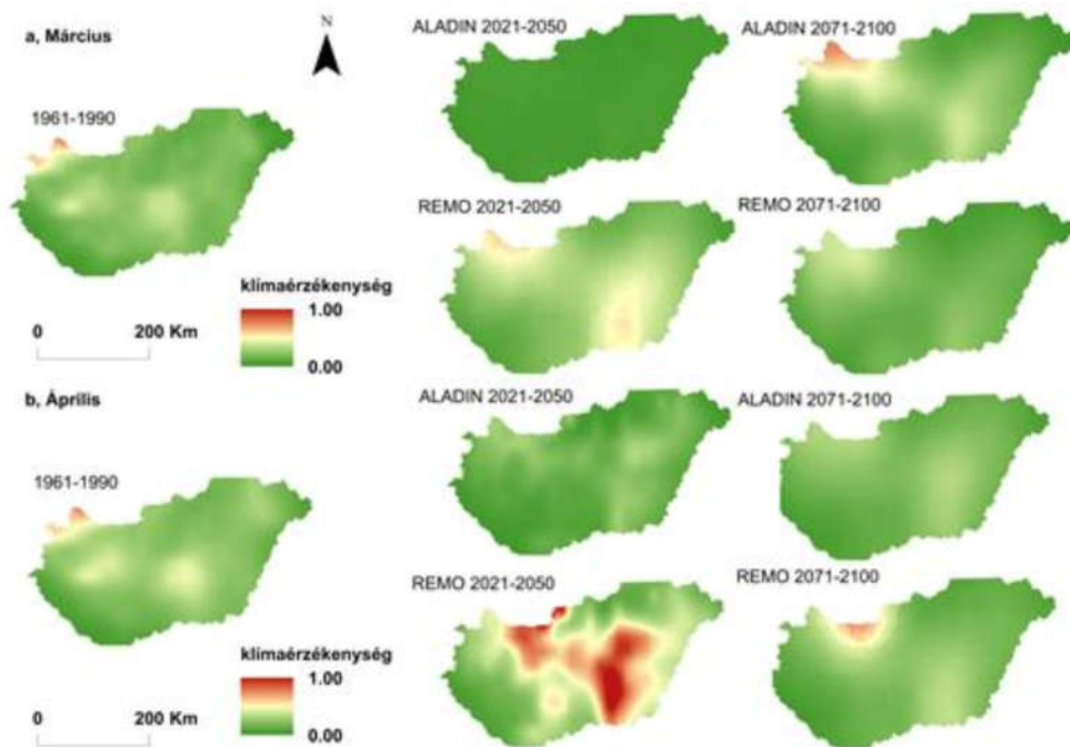
2. ábra. A klímaérzékenység (C-faktor) értékei márciusban és áprilisban 1961-1990, 2021-2050 és 2071-2100 közötti időszakban, az ALADIN és a REMO regionális klíma modell szimulációk adatai alapján
