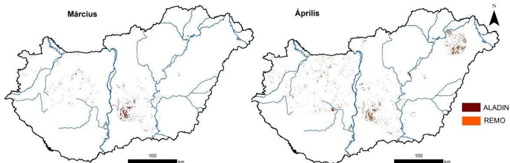
5. ábra. A szélerózió érzékenység szempontjából kiemelt jelentőségű (hot spot) területek márciusban és áprilisban az ALADIN és a REMO regionális klíma modell szimulációk adatai alapján
