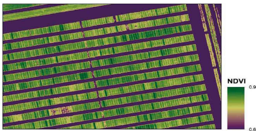
4.9 ábra Fajtaismétlődés a kísérlet északkeleti blokkjában.
