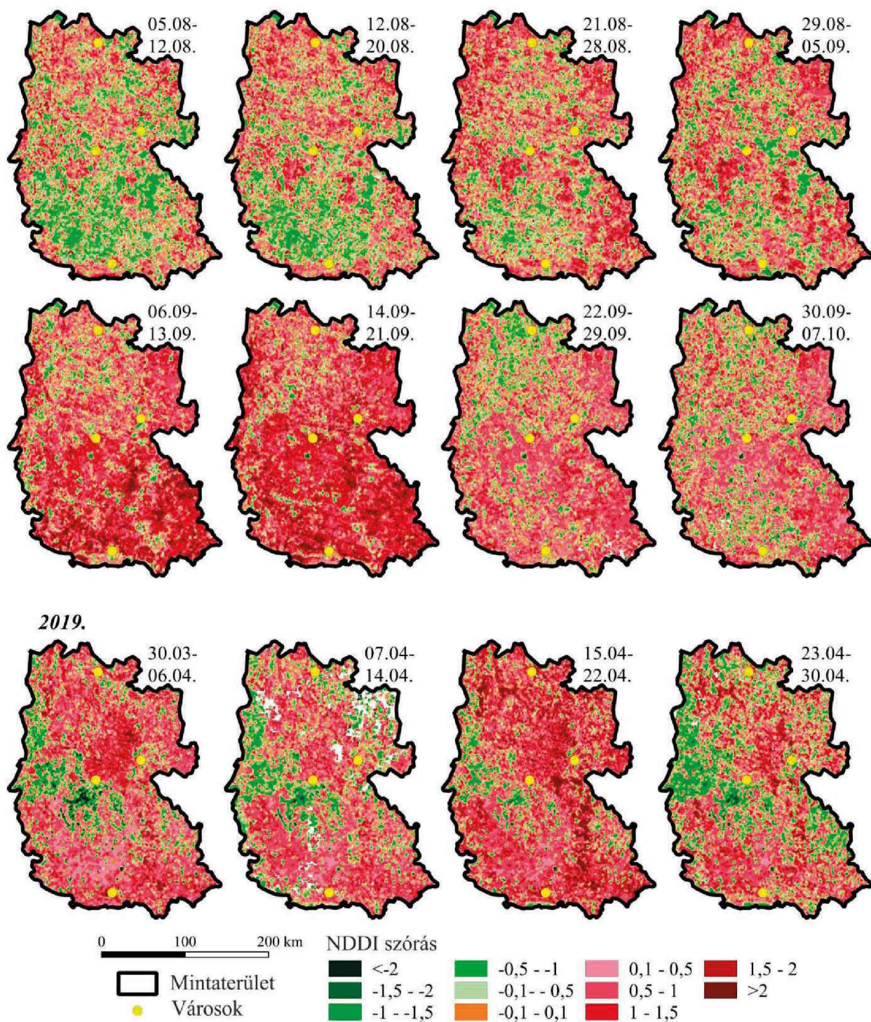
4.4. ábra Standardizált NDDI térbeli elemzése 2018-2019-ben
