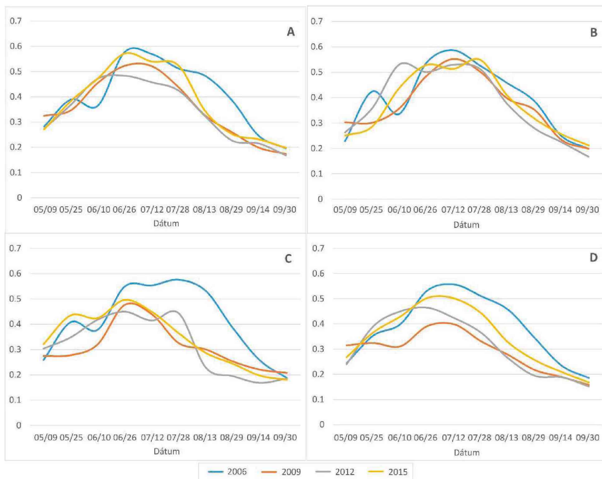
4.7 ábra A 16 napos kompozit EVI index képekből rajzolt biomassza görbék alakulása tájtypusok szerint a LUCAS adatbázis kukorica parcella pontjaira (A: Bácska; B: Dunamente; C: Duna-Tisza köze; D: Tiszántúl)
