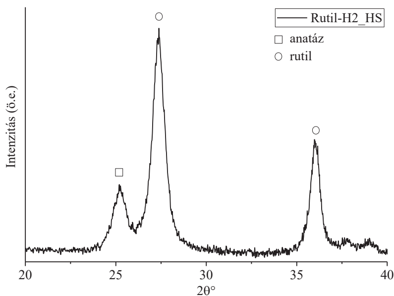
3. ábra: A Rutil-H2_HS titán-dioxidról készített XRD felvétel
