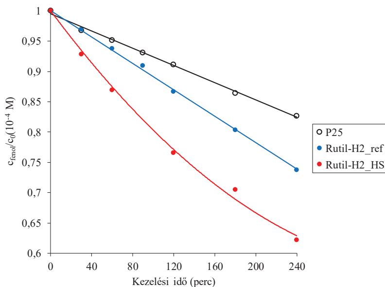
4. ábra: A fenol fotokatalitikus bontásának eredményei
